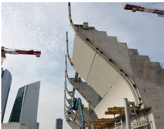
Montage des éléments préfabriqués par VINCI Construction France, en surface des gradins de tribunes de l'Arena Nanterre-La Défense.
